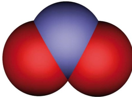
Slika 2.5 Prikaz molekule dušikovog dioksida (URL 9)
