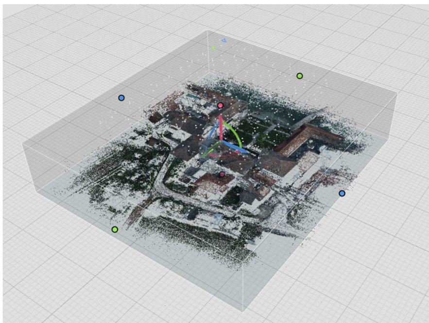
Slika 5.8. Oblak točaka nastao poravnanjem snimaka iz zraka
