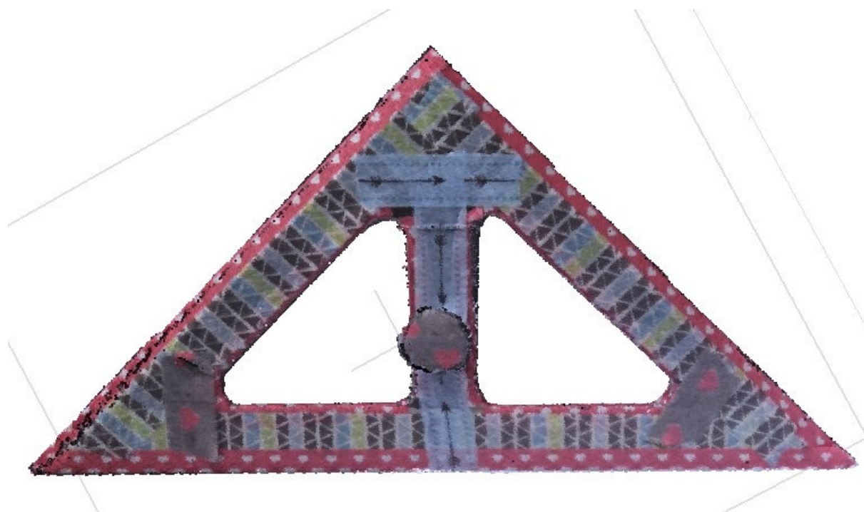
Slika 54. Oblak točaka
