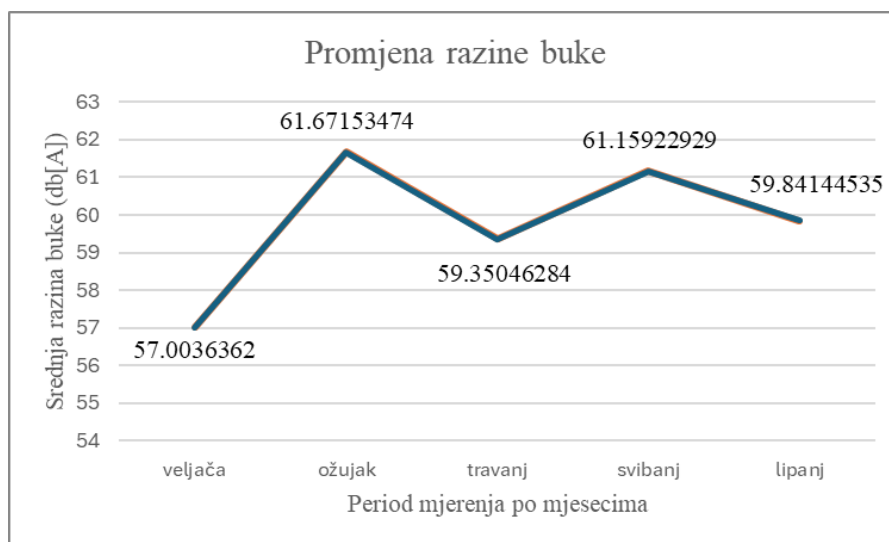
Slika 5.1. Promjena srednje vrijednosti razine buke kroz mjesece
