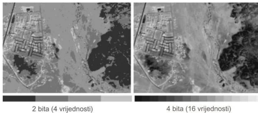
Slika 4. Prikaz različitih radiometrijskih rezolucija (modificirano prema URL 12)
